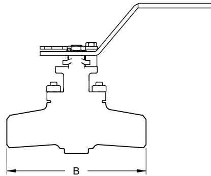
ASME CLASS 300
